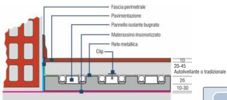
Sezione massetto
